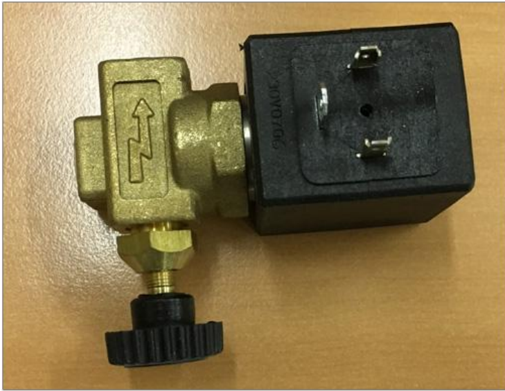
481 Клапан с регулятором Sama 150/R 1/4 "F F (для гладильных столов)
