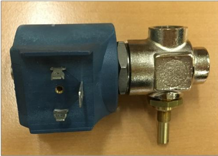
405.24 Клапан Семе ESQ 9922 1/4 "FF (для гладильных столов)
